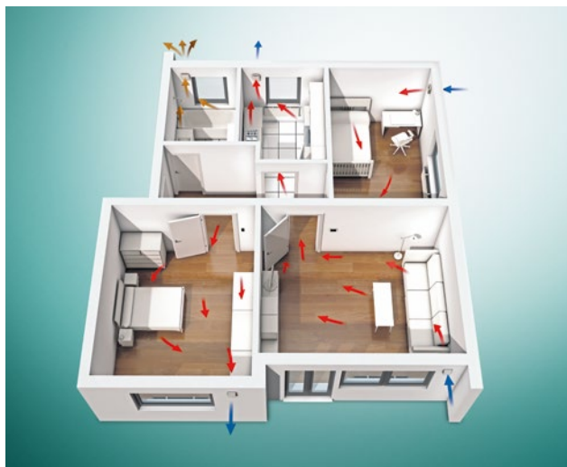
Primer sistema z recoVAIR VAR 60
