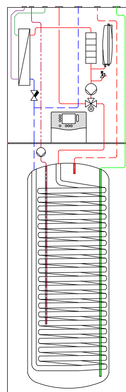
Hidravlične podrobnosti
